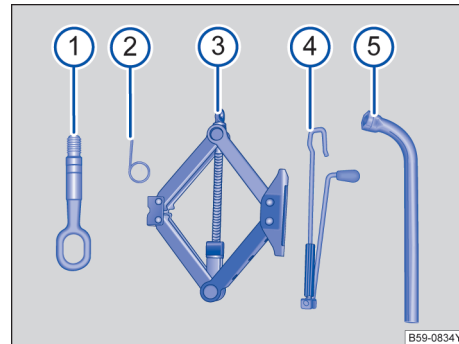
图 186 随车工具的组件
