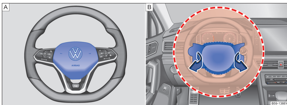
图 36 驾驶员前部安全气囊的安装位置和膨胀范围
