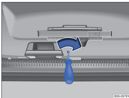
图 67 行李厢盖应急解锁
