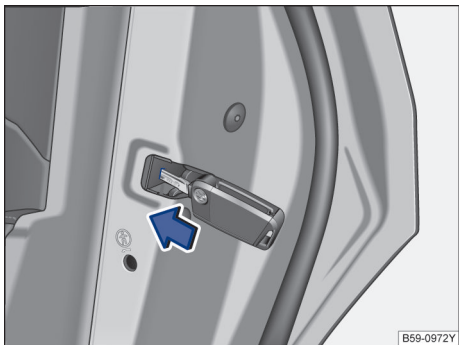
图 58 车门应急上锁装置及汽车钥匙
