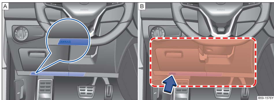
图 40 驾驶员侧：膝部安全气囊安装位置及作用范围
