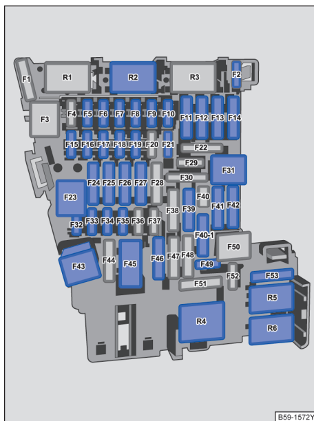
图 190 仪表板中：保险丝分配
