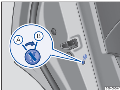
图 54 在左后车门中：儿童安全锁 (A) 已关闭、(B) 已接通
