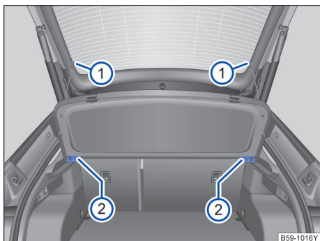
图 174 拆卸和安装行李厢盖板
