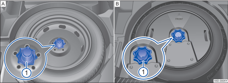
图 208 行李厢内：备用车轮固定手轮（类型 A 和类型 B）
