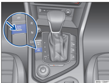
图 140 在中控台：自动驻车功能按钮
