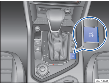
图 110 启停系统按钮
