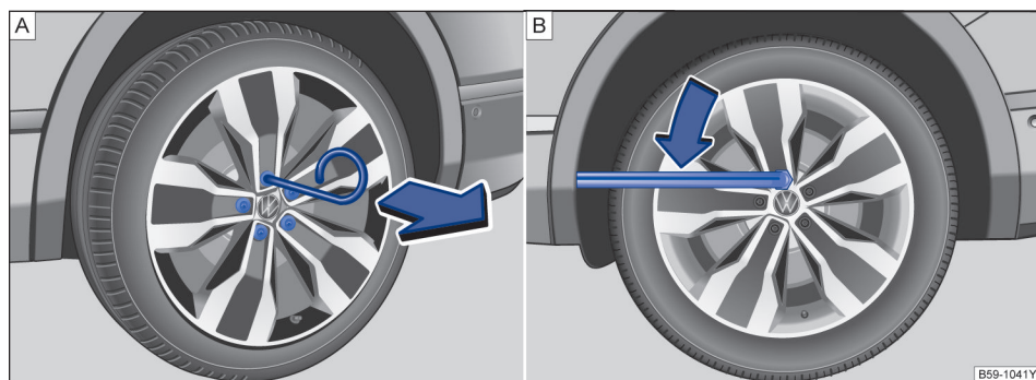
图 212 A 从车轮螺栓上拔下盖罩 B 更换车轮：松开车轮螺栓
