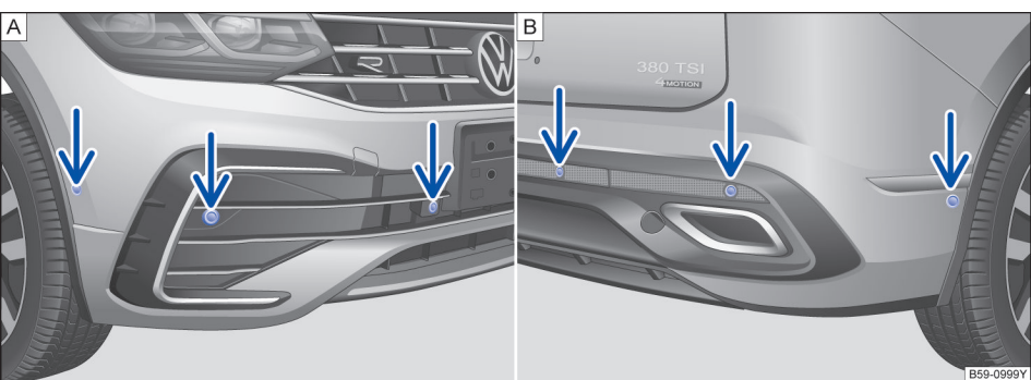
图 142 前后保险杠：泊车雷达系统超声波传感器
