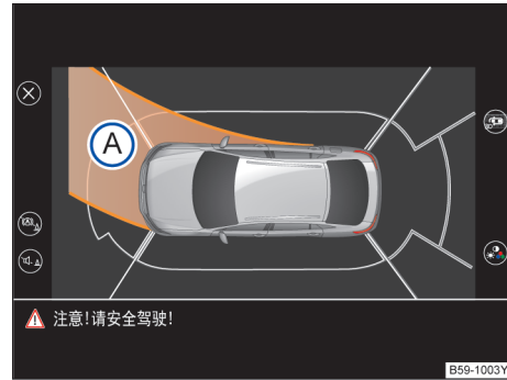
图 146 泊车雷达系统显示屏：施加转向时汽车行驶路径显示模式
