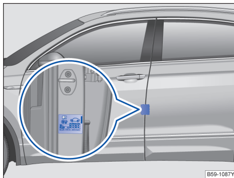
图 211 驾驶员侧中间门柱上: 胎压标签(或者在油箱盖的内侧)
