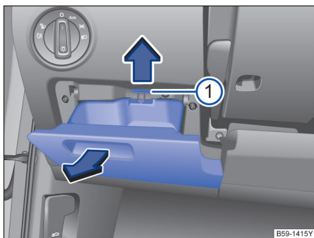
图 189 在驾驶员侧仪表板上：保险丝盒盖板
