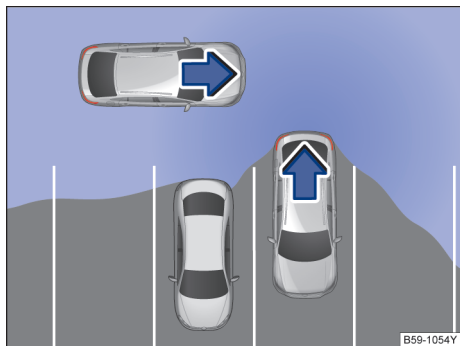
图 137 驶出车位辅助原理图：车辆驶出停车位时的车后左右两侧监控范围
