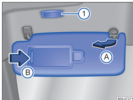
图 100 遮阳板
